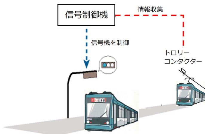
図-57 電車優先信号
